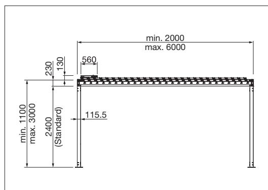
TP6500 Zijaanzicht
